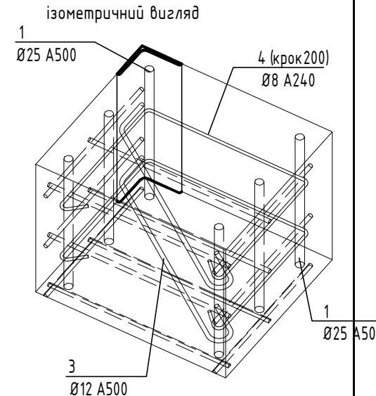
Деталь А
