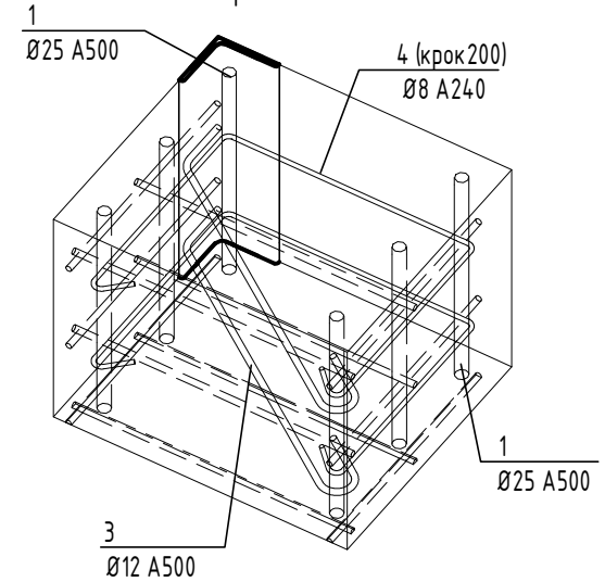
Деталь А
