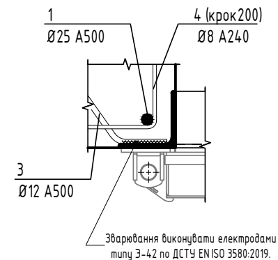
деталь А
