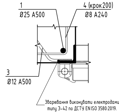
деталь А
